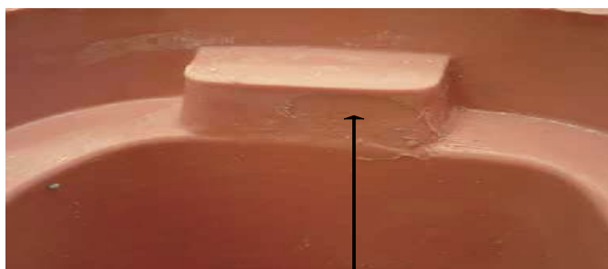
缩痕
